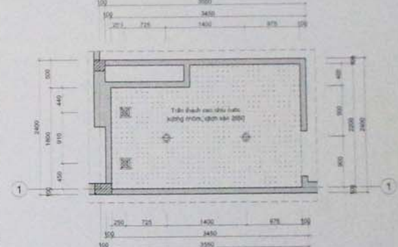
MẶT BẰNG TRẦN WC2
