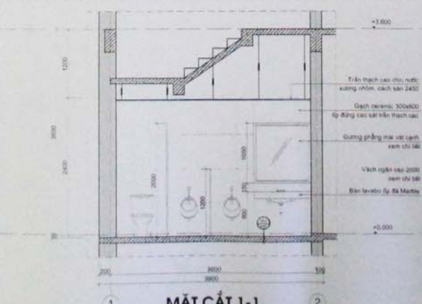
MẶT CẮT 1-1
