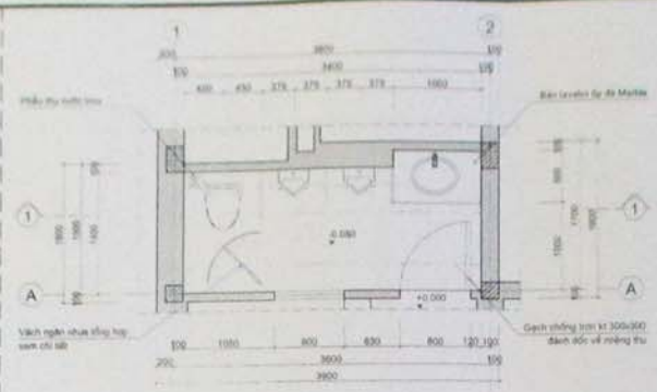
MẶT BẰNG WC1
