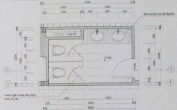
MẶT BẰNG WC2
