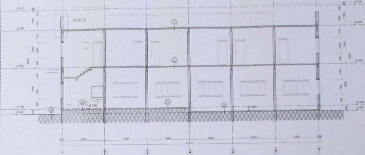
MẶT CẮT 1-1
