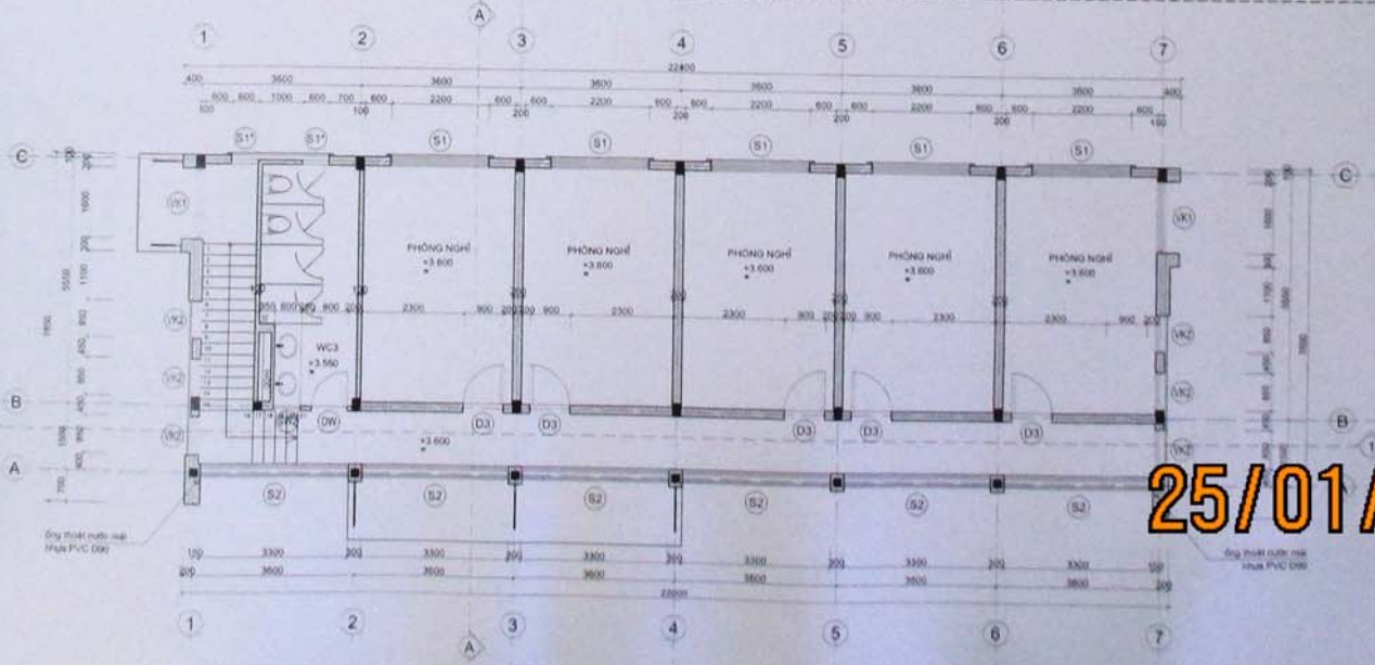
MẶT BẰNG TẦNG 2
