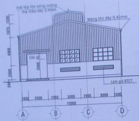
MẶT ĐỨNG TRỰC 1-6
