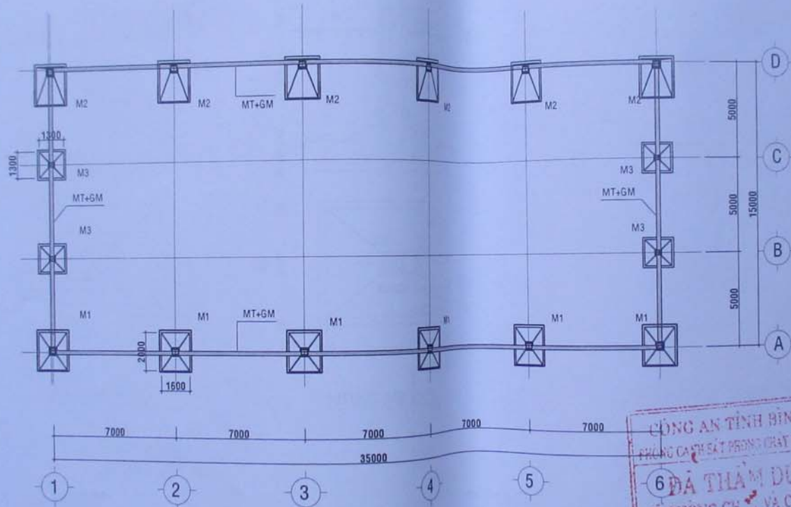
MẶT BẰNG MÓNG
