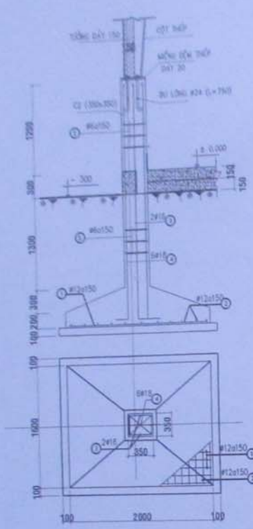
MÓNG M1 (6CK)
