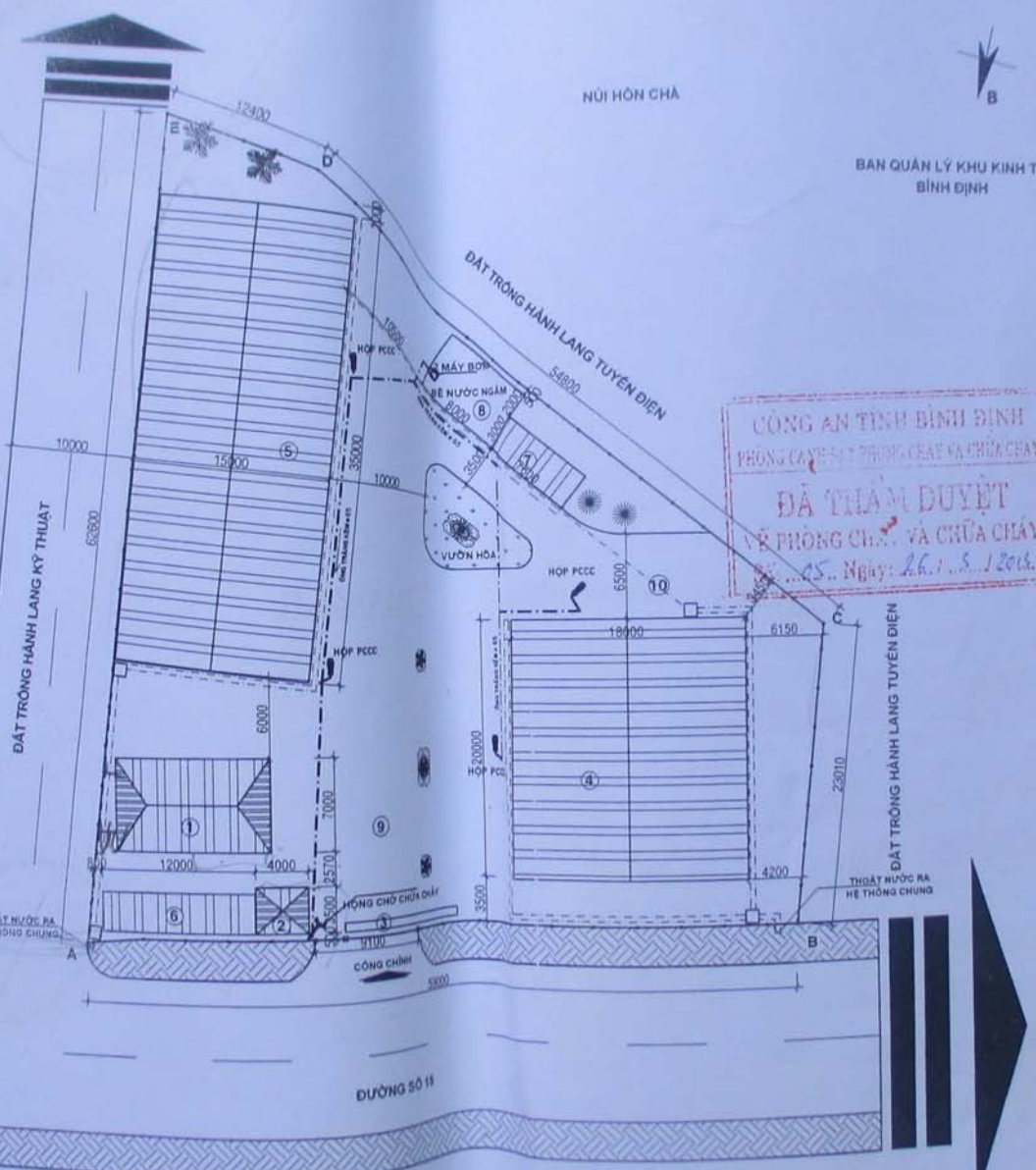
MẶT BẰNG QUI HOẠCH TỔNG THỂ TL: 1/200
