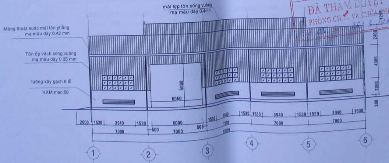
MẶT ĐỨNG TRỰC 1-6
