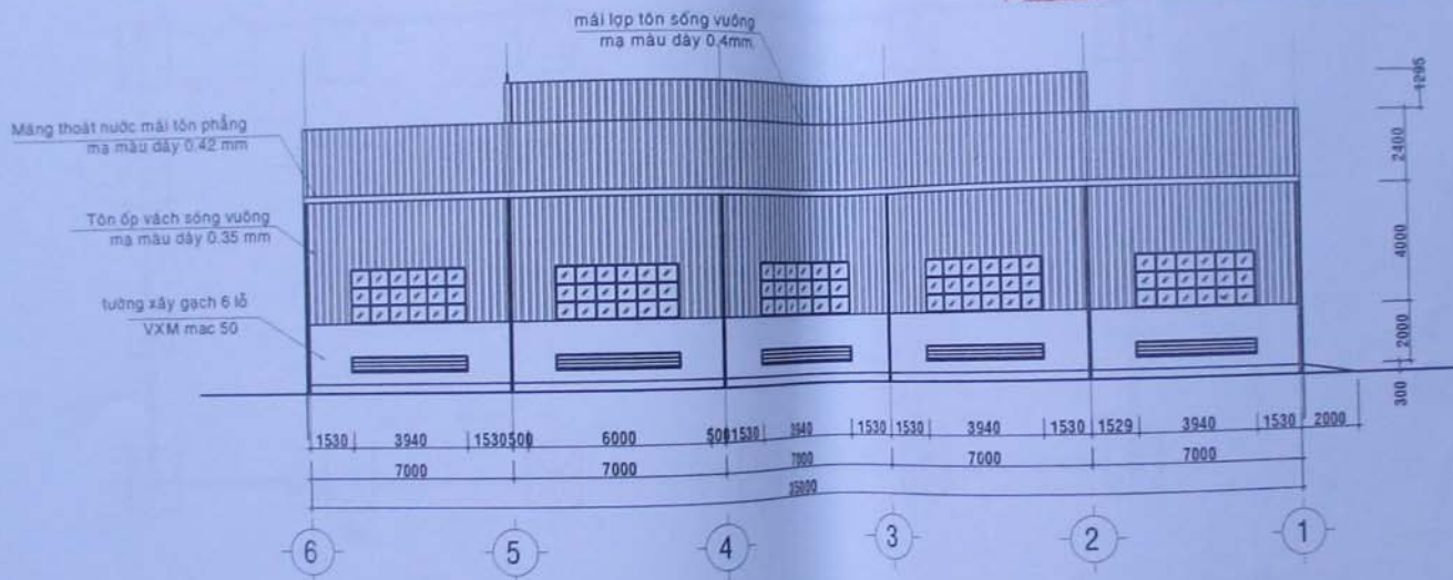
MẶT ĐỨNG TRỤC 6-1
